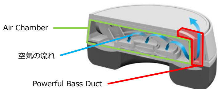
重低音再生を実現するハウジング構造
